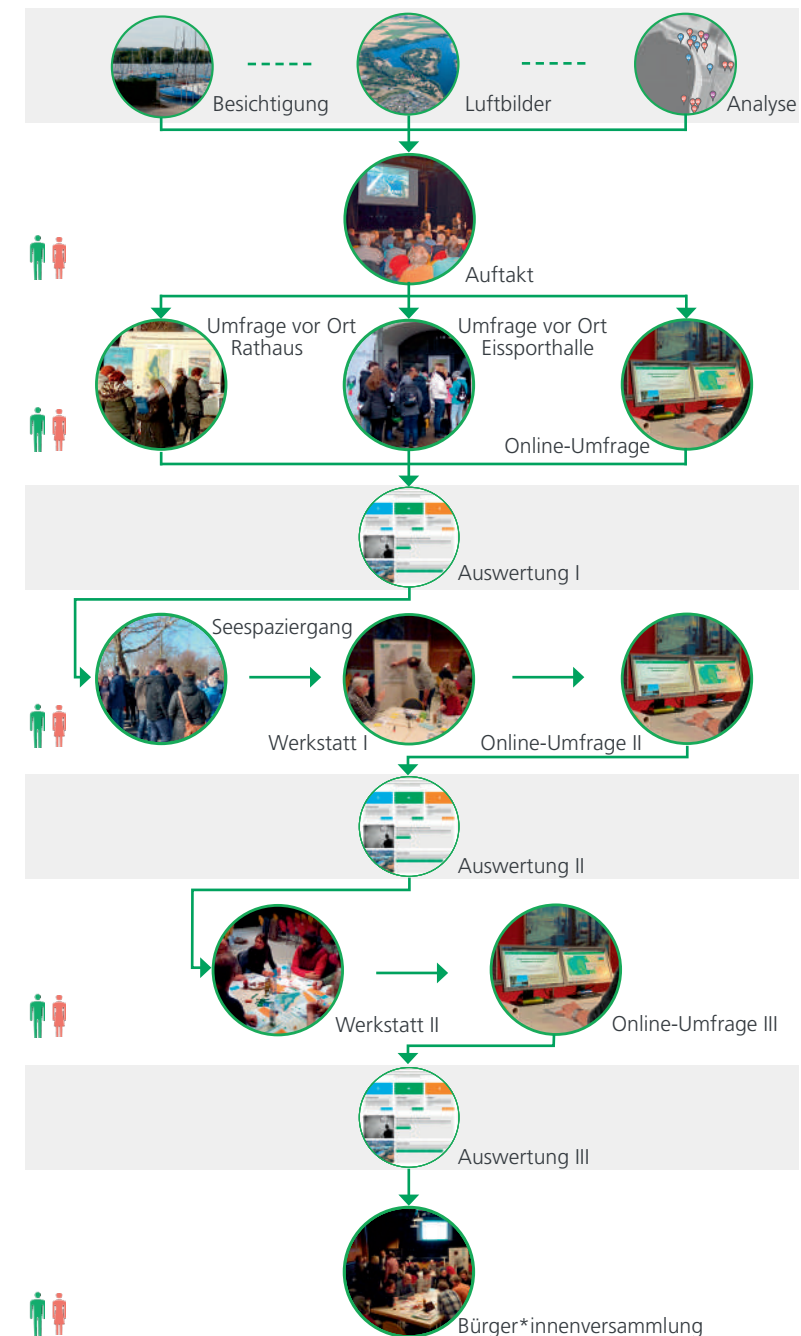
Prozessdiagramm Öffentlichkeitsbeteiligung
