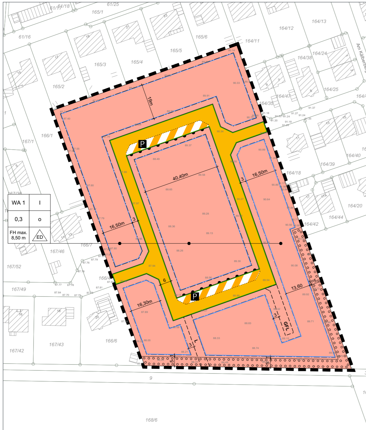
Planzeichnung zum Bebauungsplan Geltungsbereich A
